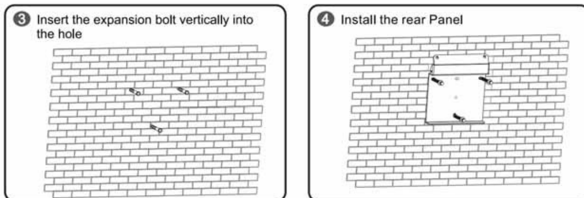
Figura 2-8 Schema dell'installazione del pannello posteriore dell'inverter
